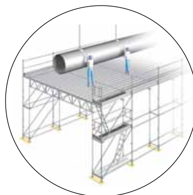
STAR stillas og bærende gitterdrager for stillasgulv
